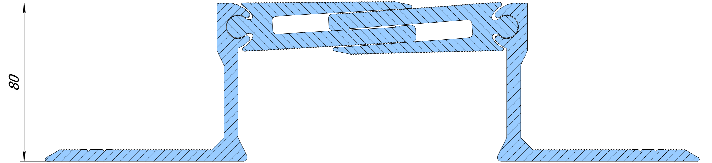
Dewmark Heavy SV 45/135/80
