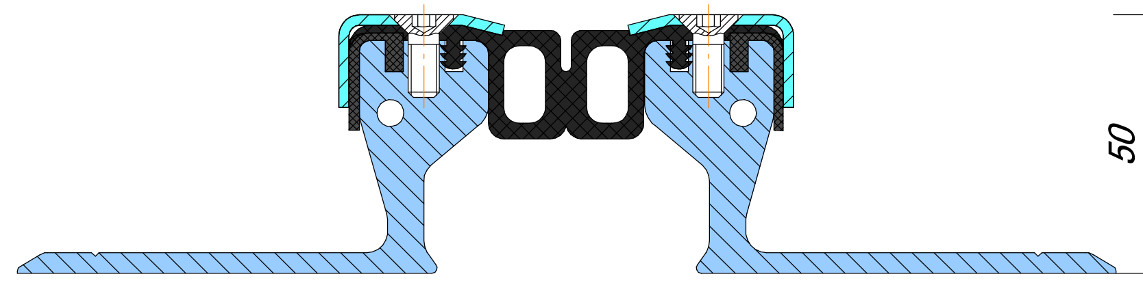
Dewmark Hydro WR 73/50/50/S
